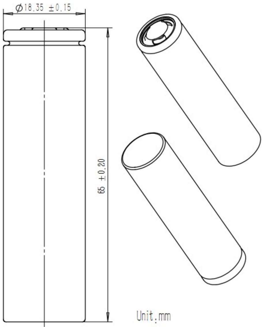
附图 1: 规格尺寸外形图
