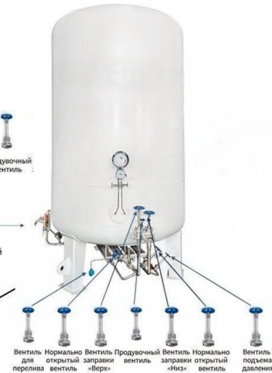
Предохранительный клапан
